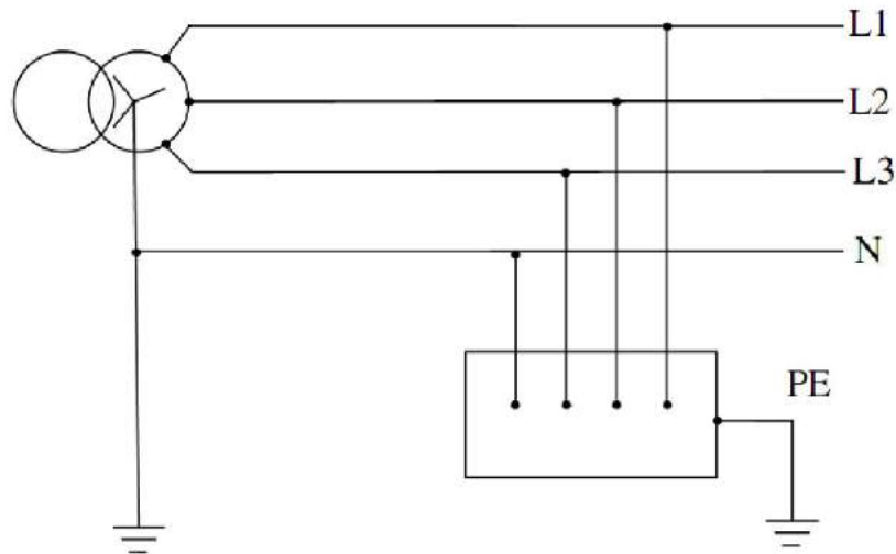
Hình 2.2 - Sơ đồ TT
