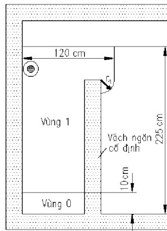
b - Hình chiếu cạnh (có vách ngăn cố định và bán kính xác định khoảng cách nhỏ nhất từ đầu phía trên của vách ngăn)
