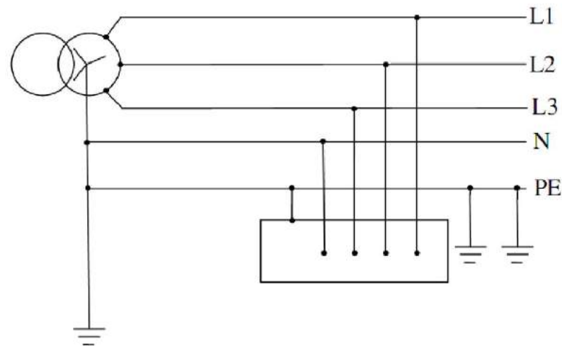
Hình 3.3 - Sơ đồ TN-S
