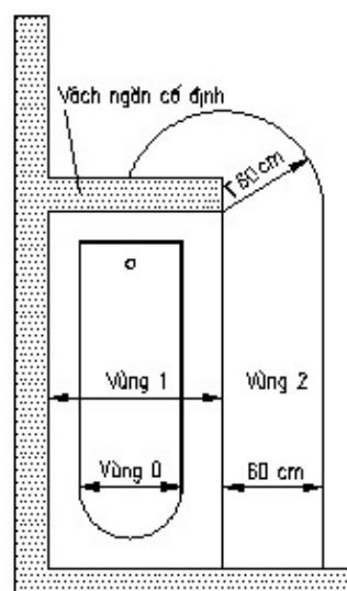
c - Hình chiếu bằng (có vách ngăn cố định và bán kính xác định khoảng cách nhỏ nhất quanh vách ngăn)
