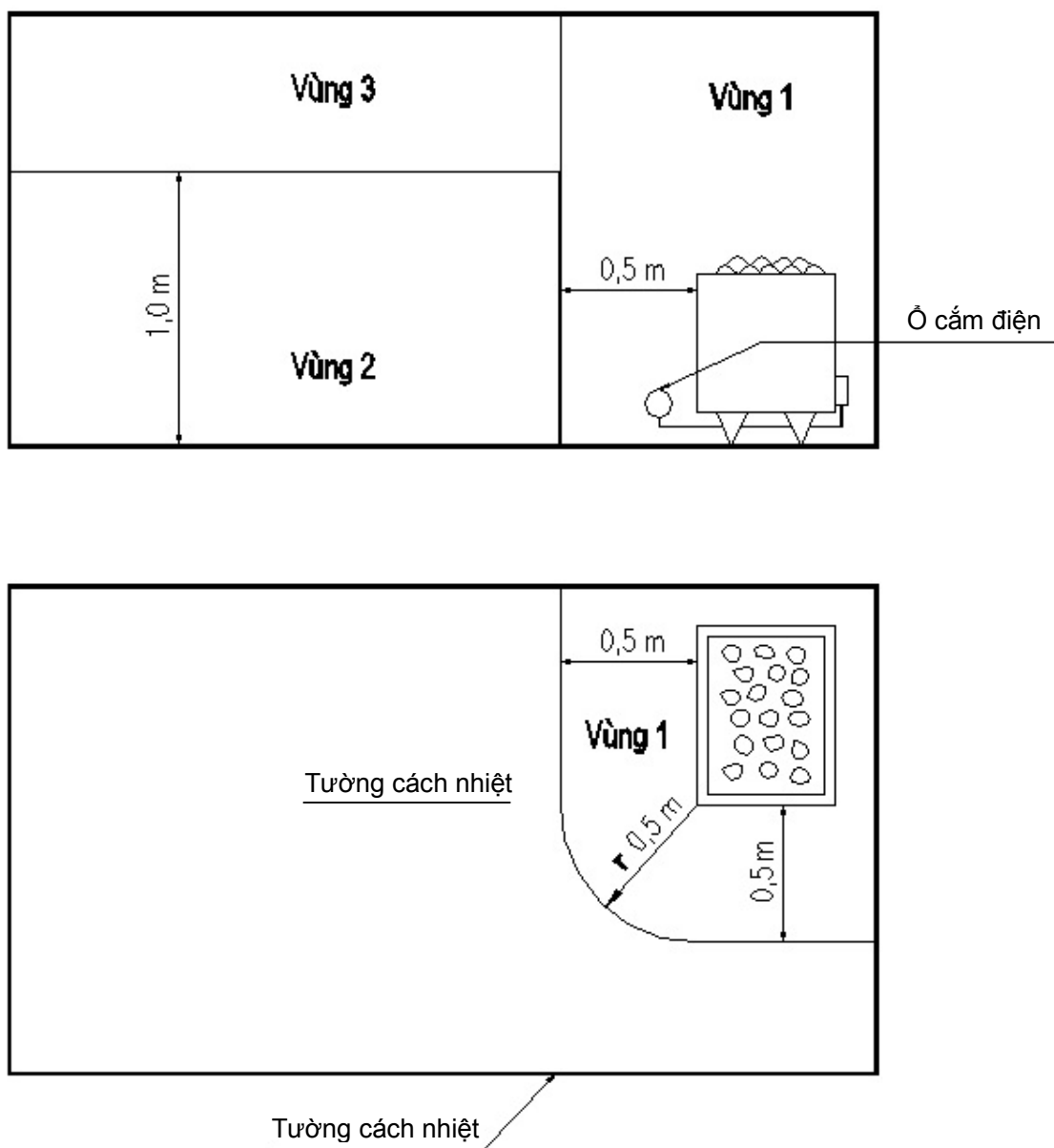
Hình N.6 - Kích thước các vùng của khu vực lân cận phần tủ gia nhiệt sinh hơi
